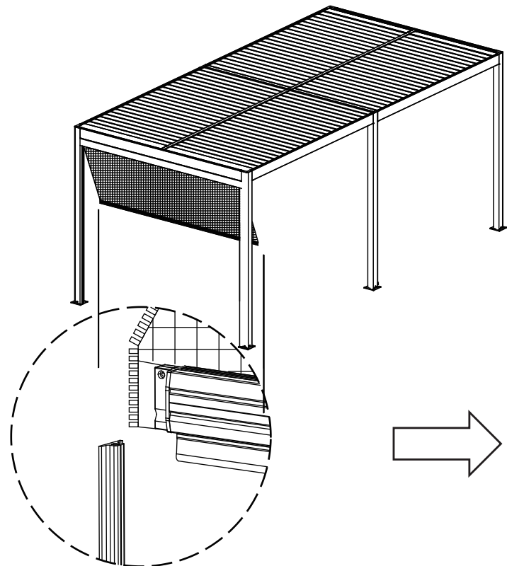
Installer le rail intérieur
