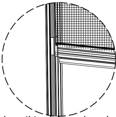
Installer le rail intérieur dans le rail arrière
