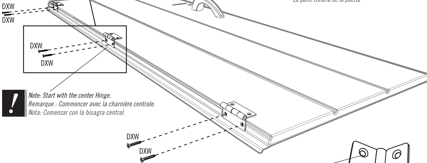
Rear of Door / La partie arrière de la porte La parte trasera de la puerta
