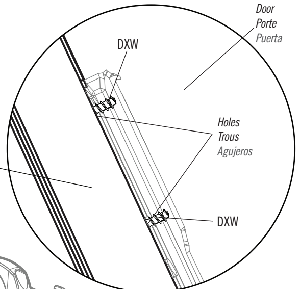
Rear of Door / La partie arrière de la porte La parte trasera de la puerta
